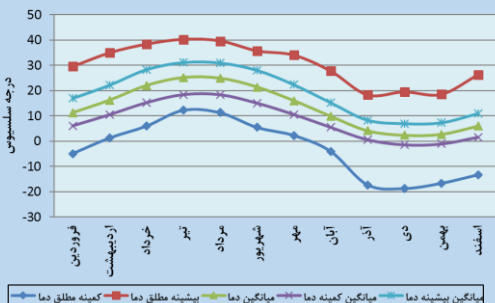
نمودار رژیم ماهانه دمایی در شهرستان راز و جرگلان (۱۳۸۵-۱۳۹۷)
