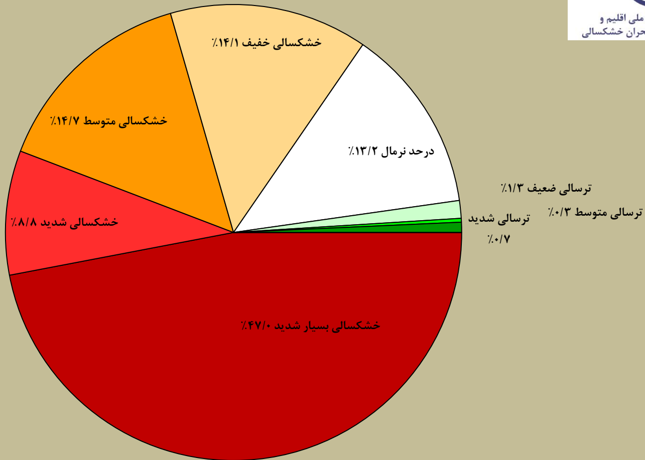
درصد مساحت تحت تاثیر خشکسالی براساس شاخص SPEI دوره ده ساله تا پایان مرداد ماه ۱۴۰۱ در سطح استان خراسان شمالی
